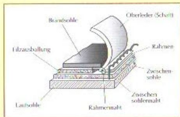
Abb.: Querschnitt eines rahmengenähten Szabőr-Schuhs mit doppelter Sohle.
